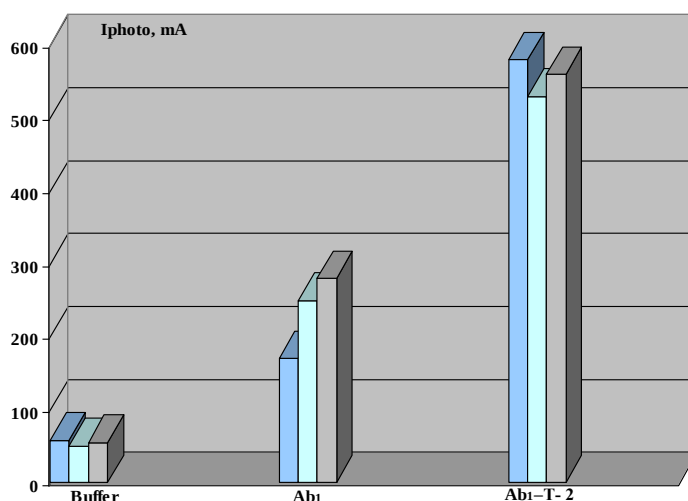
Рис. 5. Зміни фотоструму фоторезистора після додавання буфера, специфічних антитіл ( Ab_1 ) та утворення комплексу Ab_1 -Т-2 мікотоксин
