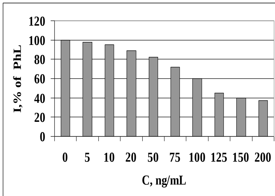
Рис. 7. Залежність сигналу імуносенсора (інтенсивність сНПКФЛ) від концентрації T2-мікотоксину в аналізованому розчині
