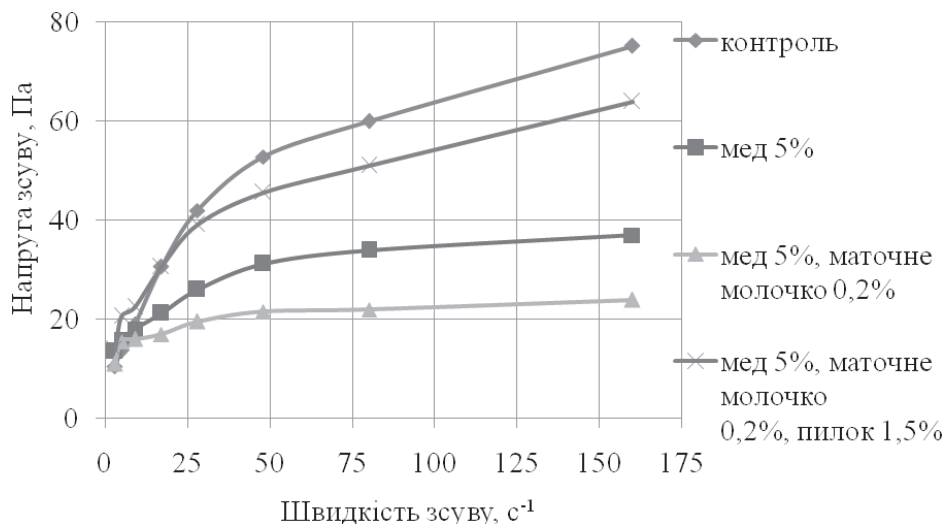
Рис. 3. Залежність напруги зсуву зразків йогурту від градієнта швидкості, c^{-1}
