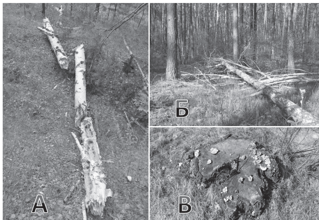
Рис. 2. Мортмаса деревної ламані берези: А) деревна ламань, утворена з сухостійного дерева; Б) деревна ламань утворена від несприятливих погодних умов; В) мортмаса пня
