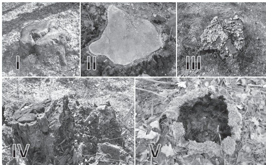
Рис. 8. Мортмаса пнів I–V класів деградації: I - свіжий пень I класу деградації після зрубання живого дерева; II - пень II класу деградації після зрубання сухостійного дерева без гілок; III - пень III класу деградації з плодовими тілами грибів; IV - трохавий пень IV класу деградації зі збереженою формою; V - залишки пня V класу деградації
