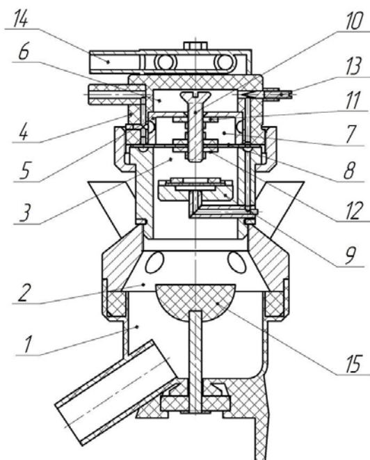
Рис. 1. Конструктивна схема колектора адаптивного доїння: 1 – пластмасовий корпус (К1); 2 – камера; 3 – стакан; 4 – камера змінного вакууму; 5 – стакан; 6 – верхня частина стакана (К3); 7 – нижня частина (К2); 8 – мембрана; 9 – клапан односторонньої дії; 10 – клапан; 11 – обмежувач; 12 – гайка; 13 – гвинт регульований; 14 – розподільник вакууму (К4); 15 – клапан.
