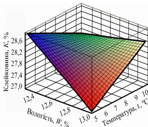
Рис. 5. Залежність вмісту клейковини від вологості зерна W та температури повітря у зерносховищі t при фіксованих значеннях факторів t_3 = 9,5^\circ\text{C} , t_{хд} = 4^\circ\text{C} , V = 10800\text{ м}^3/\text{год} .
