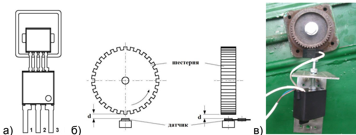
Рис. 9. Датчик кутової швидкості КМІ16/1: а) зовнішній вигляд датчика; б) розташування датчика; в) датчик на експериментальній установці.
