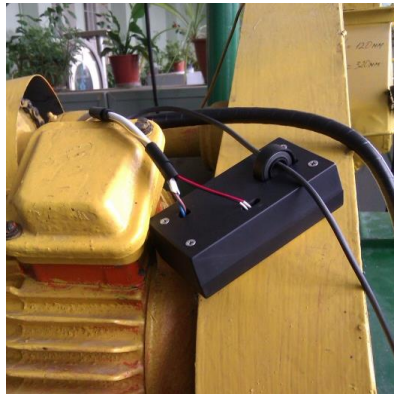
Рис. 10. Датчик струму
