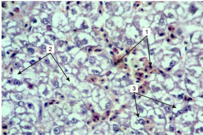
Рис. 1. Гістопрепарат печінки гусеняти віком 3 місяці за амідостомозно-гангулетеракозної асоціативної інвазії: 1 – діapedезні крововиливи, 2 – некроз гепатоцитів, 3 – гідропічна дистрофія гепатоцитів (Гематоксилін Караці та еозин, x 200)
